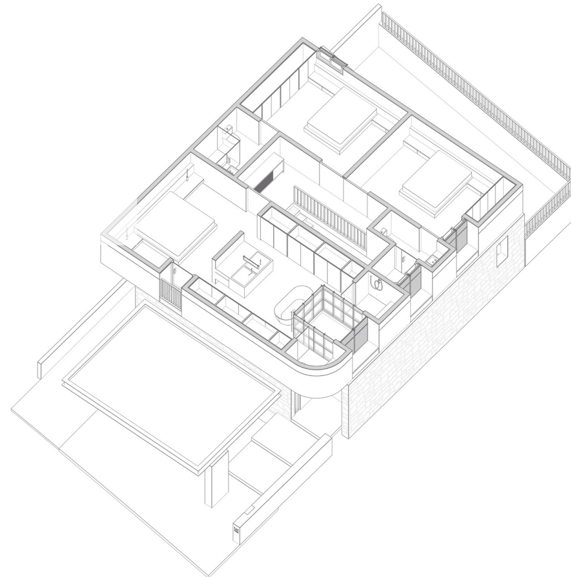
Axonométrico PA
