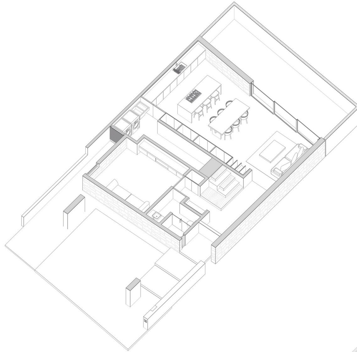
Axonométrico PB
